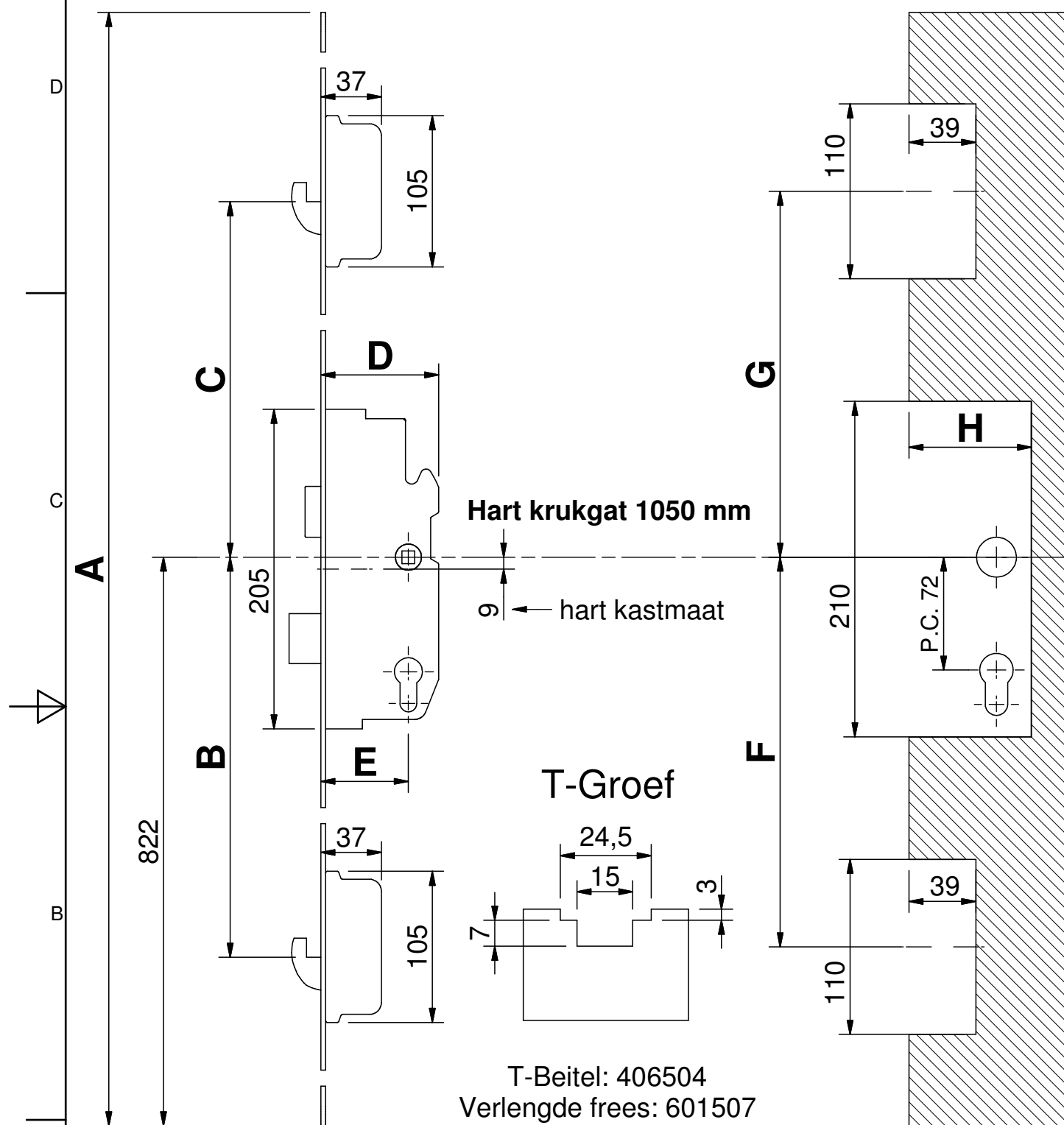
Overzicht afmetingen Sleutelbediende Meerpuntssluitingen
